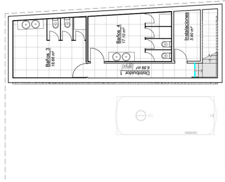
planta sótano
